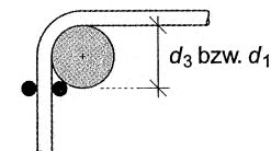
Figur 33: Schweissstellen bei gebogenen Matten
